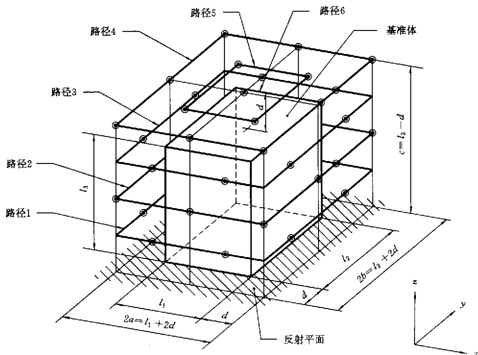
图 C5 中型机器测量表面和传声器位置(路径)示例
